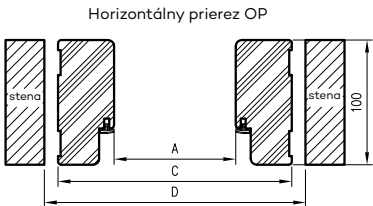
rovna zárubňa soft
