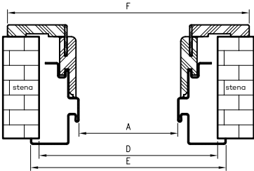
Profil zárubne
