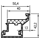
DRE profil pre dovnútra otvárateľné reverzné falcové dvere
